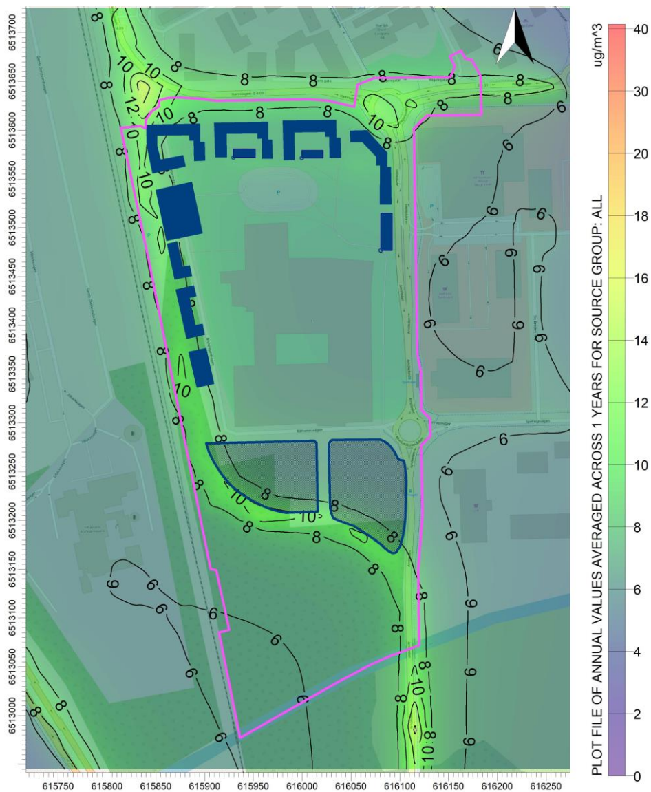
Figur 4. Framtida scenario 2040 , beräknade halter av kvävedioxid som årsmedelvärden. Planområdet markeras med lila linje.
