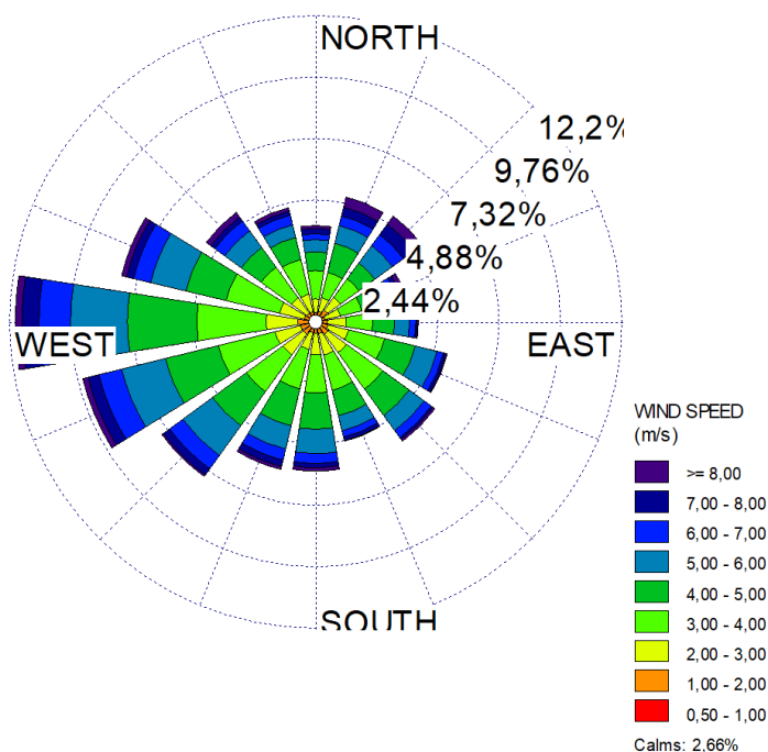
Figur 2. Vindros för meteorologiska data året 2009-2013 i Nyköping
