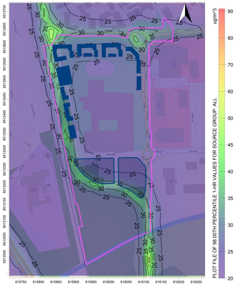
Figur 8. Framtida scenario 2040 , beräknade halter av kvävedioxid som timmedelvärden (98-percentil). Planområdet markeras med lila linje.
