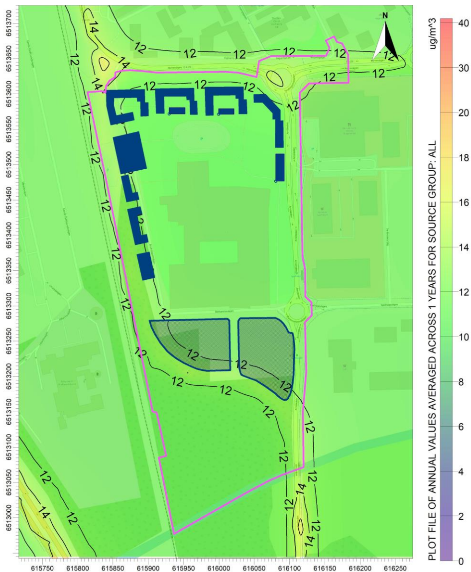
Figur 10. Framtida scenario 2040, beräknade halter av partiklar ( PM_{10} ) som årsmedelvärden. Planområdet markeras med lila linje.
