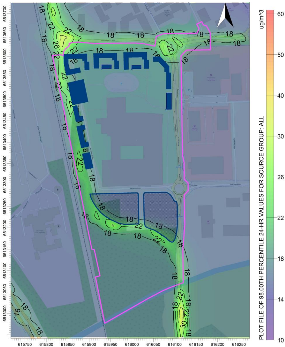
Figur 6. Framtida scenario 2040 , beräknade halter av kvävedioxid som dygnsmedelvärden (98-percentil). Planområdet markeras med lila linje.
