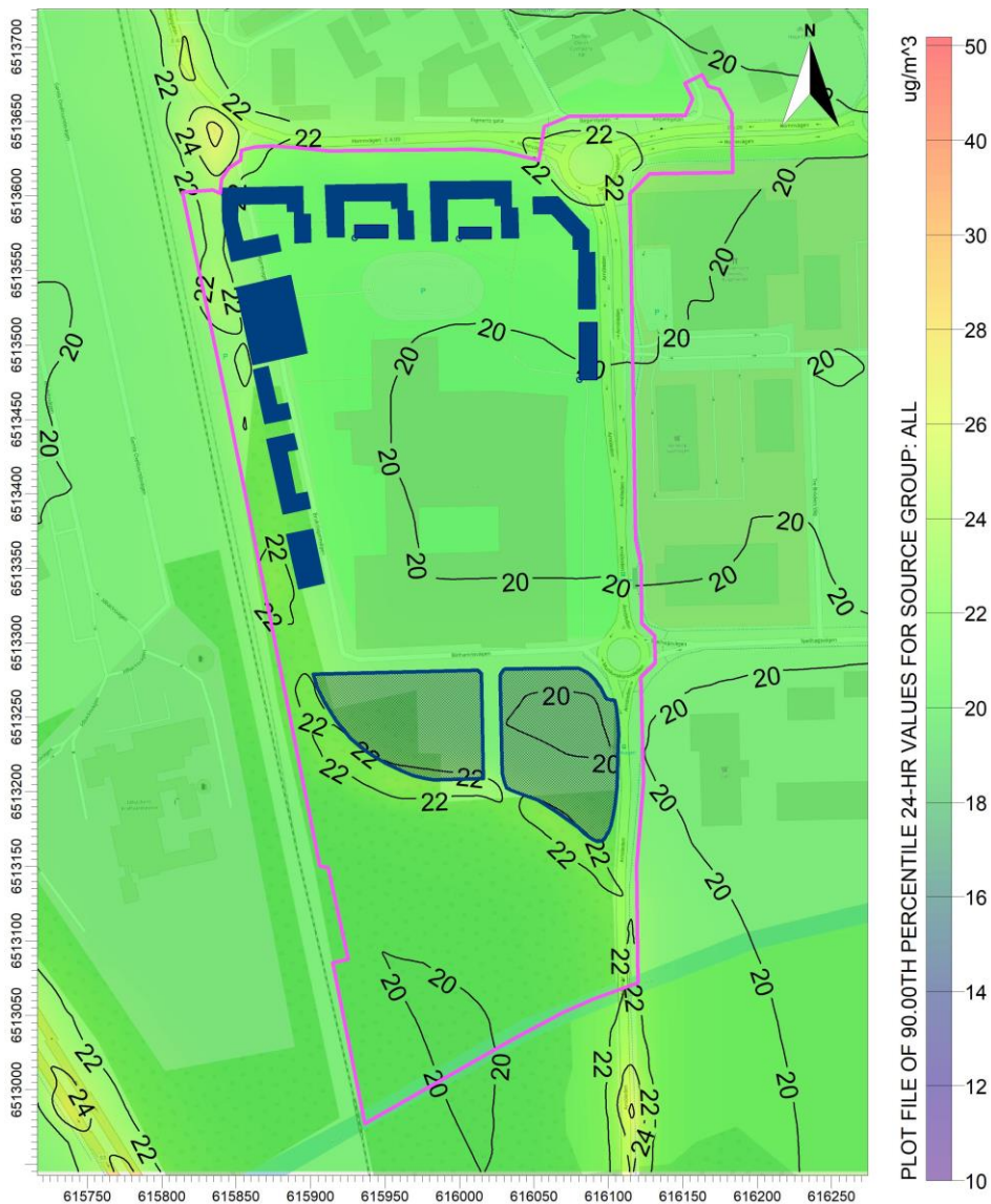
Figur 12. Framtida scenario 2040, beräknade halter av partiklar ( PM_{10} ) som dygnsmedelvärden (90-percentil). Planområdet markeras med lila linje.
