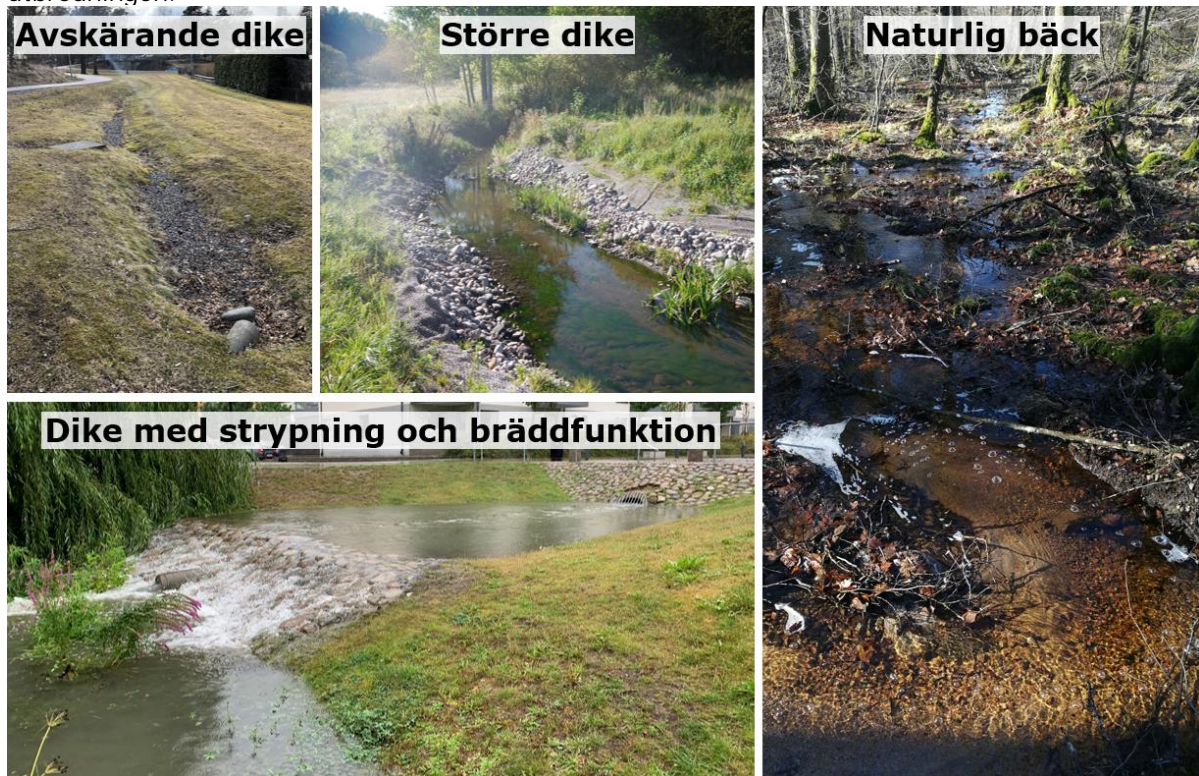
Figur 24 Olika typer av diken (Foto: Ramboll)
