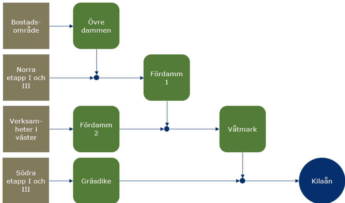
Figur 23 Dagvattensystemets uppbyggnad
