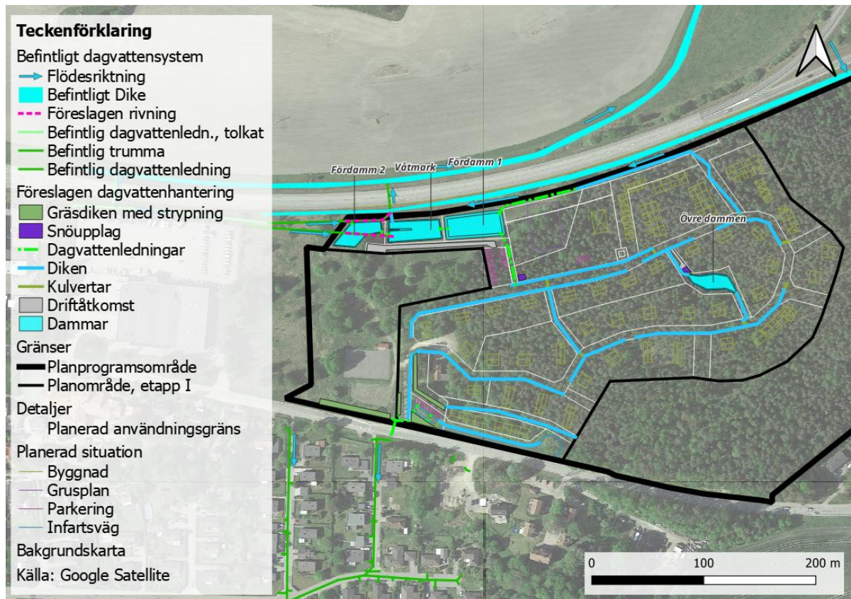
Figur 20 Föreslagen dagvattenhantering
