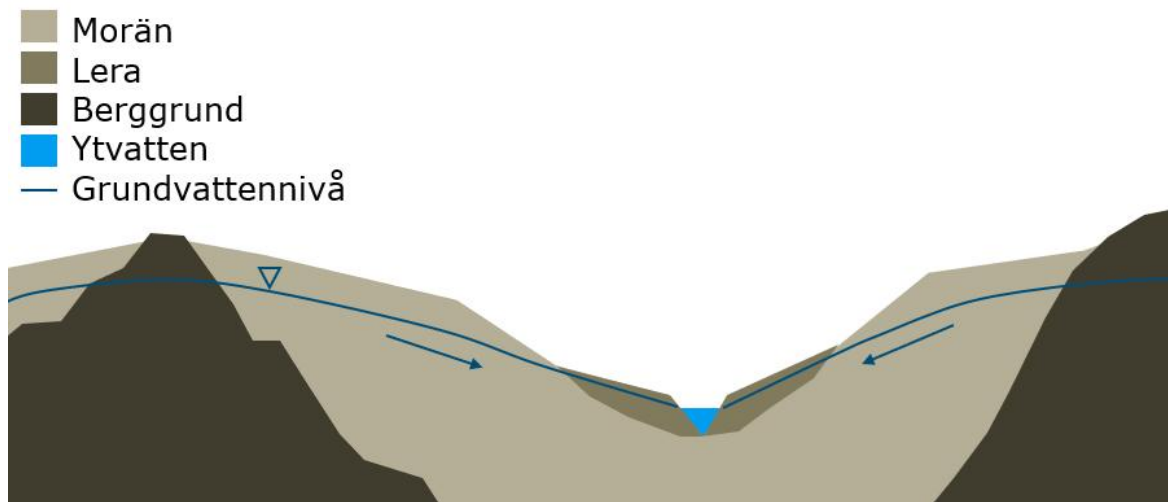
Figur 7 Principiellt: grundvattenflöde och grundvattennivå i kuperad terräng med morän, berg och lera, sektion ytvatten
