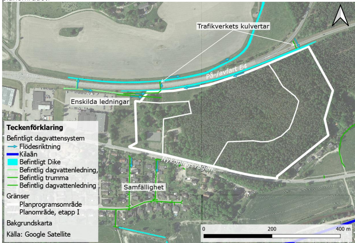
Figur 9 Befintliga dagvattenledningar
