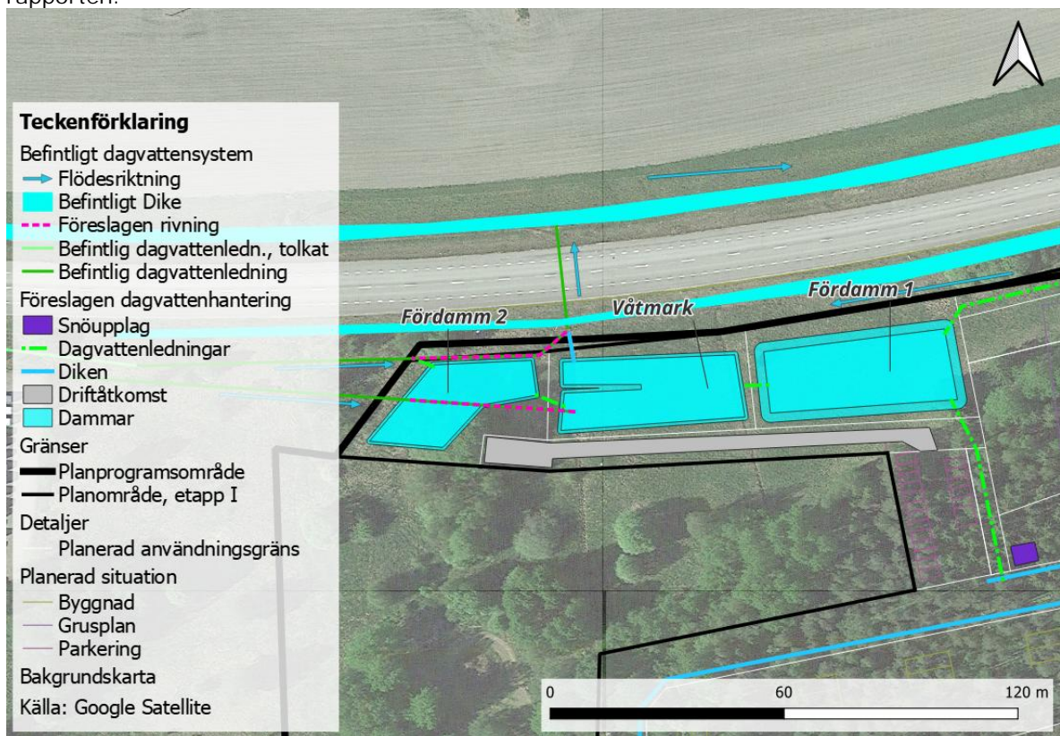
Figur 21 Detalj fördamm 1, fördamm 2 och våtmark
